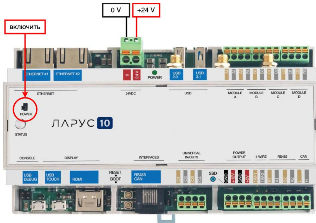
Рисунок 41 – Подключение устройства
