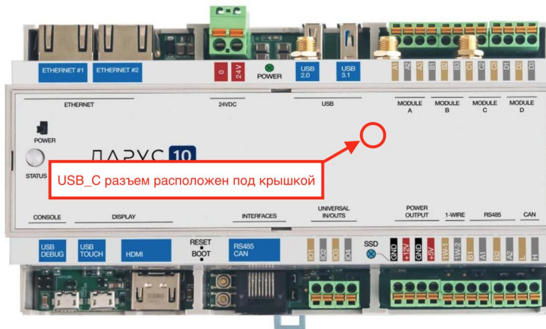
Рисунок 43 – Расположение USB-C
