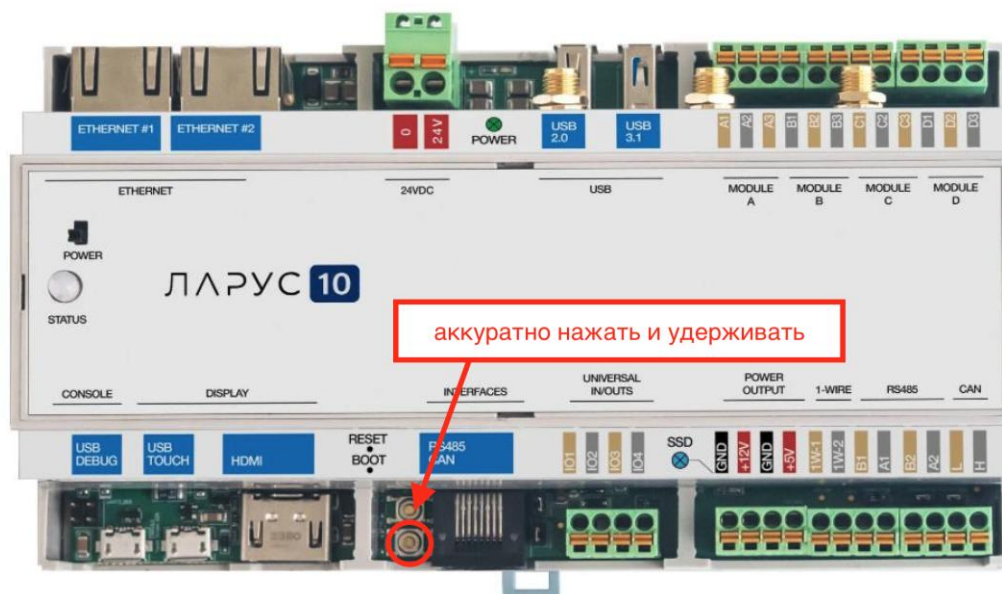
Рисунок 44 – Запуск питания
