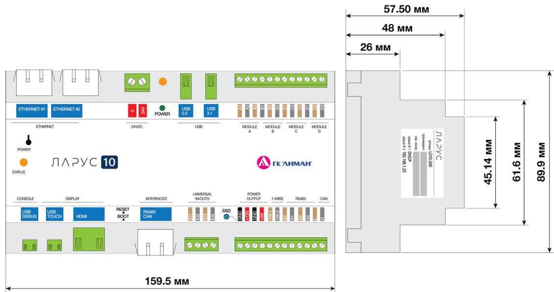
Рисунок 35 – Габариты устройства
